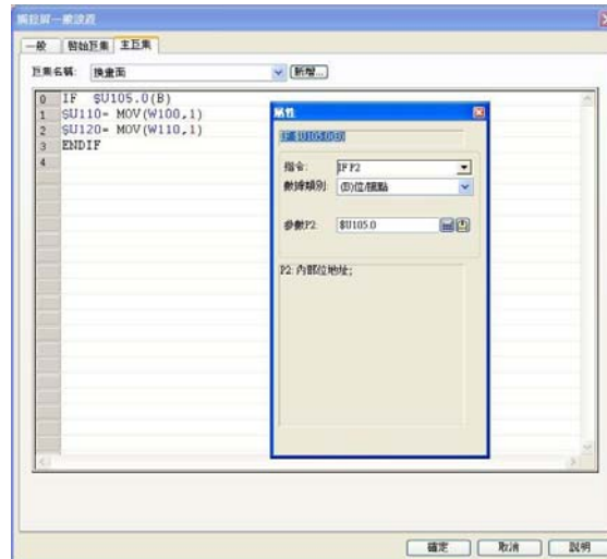
觸控屏一般設置功能_主巨集
