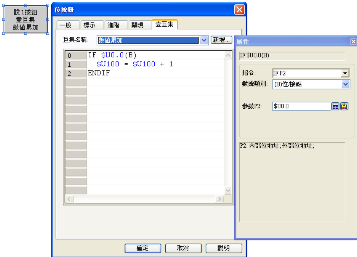
位按鈕屬性_壹巨集設置
