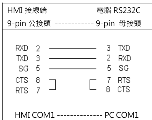
電腦和觸控屏的傳輸線接線圖
